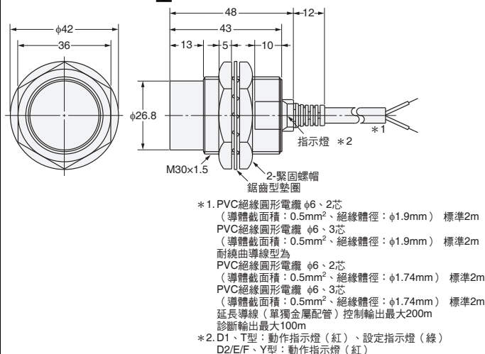
■13 E2E-X20MD□型/E2E-X18ME□/F□型 E2E-X18MY□型
