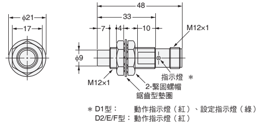
圖19 E2E-X5MY□-M1型
