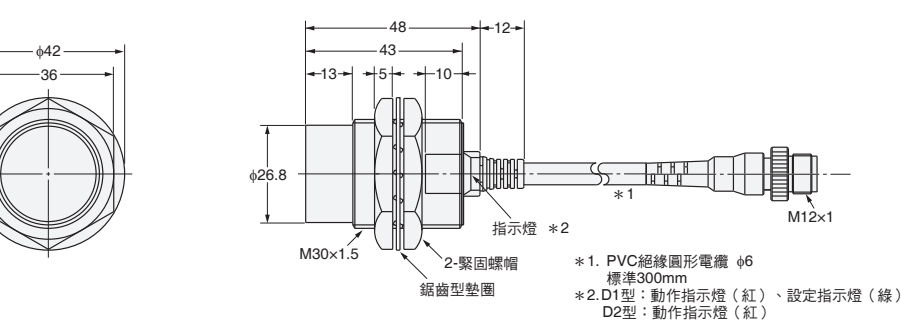
圖33 E2E-X20MD1-M1GJ型 E2E-X20MD1-M1TGJ型 E2E-X20MD□-M1TGJ-US型
