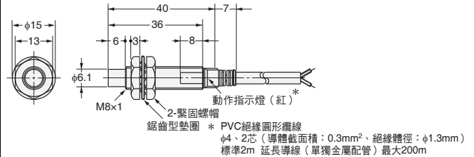
圖6 E2E-X8MD□型 E2E-X5ME□/F□型
