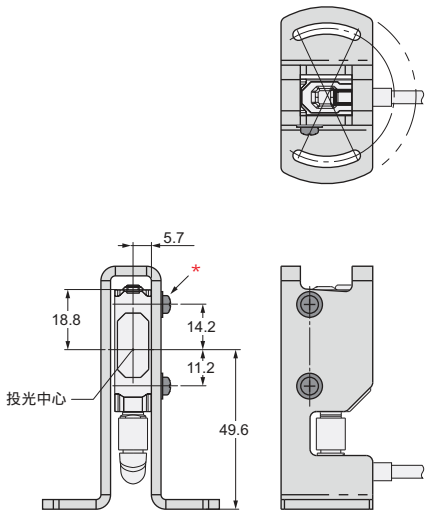
安裝感測器時的尺寸 (例：E3AS-F1500□)
