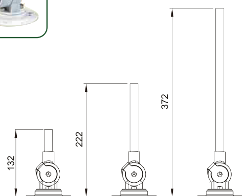
BTL 盤座尺寸圖 (mm)
